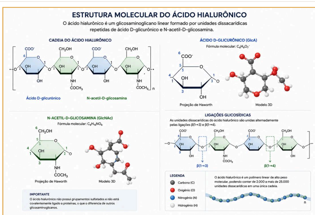
Figura 3. Arquitetura molecular do ácido hialurônico: as duas unidades monossacarídicas em projeção de Haworth e modelo tridimensional, com as ligações glicosídicas alternadas \beta(1 \rightarrow 3) e \beta(1 \rightarrow 4) . Os grupos que aparecem na cadeia — carboxila ( COO^- ), hidroxila (OH) e acetamido ( NH-COCH_3 ) — são os que dão ao HA sua avidez por água e, no passo seguinte, os pontos onde a reticulação acontece.
